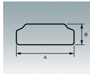
M0000804 Découpe HDMI Outils de poinçonnage
