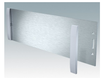
M5700613 Kit de plaque avant (3/3H) Aluminium Anodisé mat 219,5x2x65,1mm
