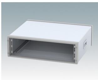
M6019325 INSTRUMET 19" 3Ux450mm Aluminium Gris clair/gris fenêtre RAL 7035/7040 157x516x450mm
