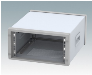
M6010305 INSTRUMET 10.5" 3Ux350mm Aluminium Gris clair/gris fenêtre RAL 7035/7040 157x303x350mm
