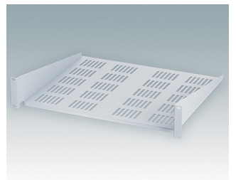
M6119285 Etagère 2U pour rack 19" Acier doux CR4 Gris clair RAL 7035 88,1x482,6x400mm
